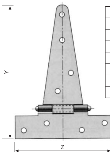
Bisagra atornillar AISI 304
